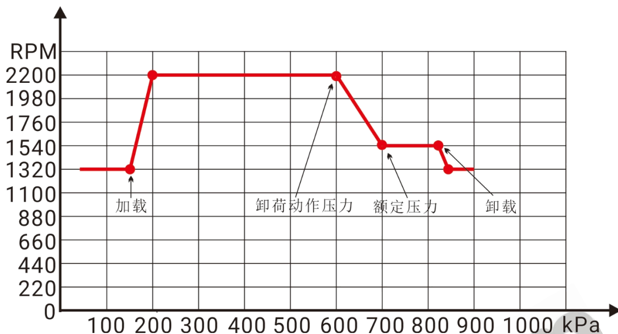
图2 转速-压力曲线图
