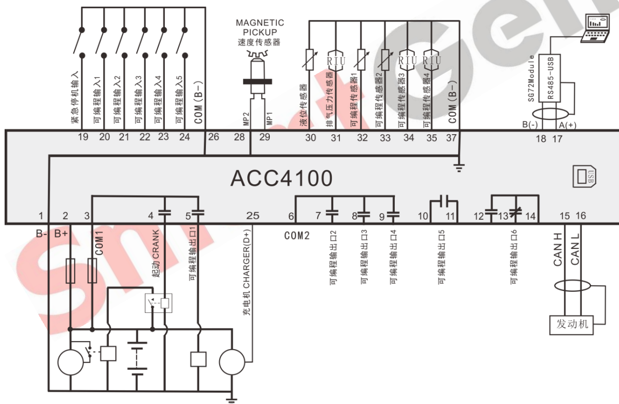
图8 ACC4100 典型应用图
