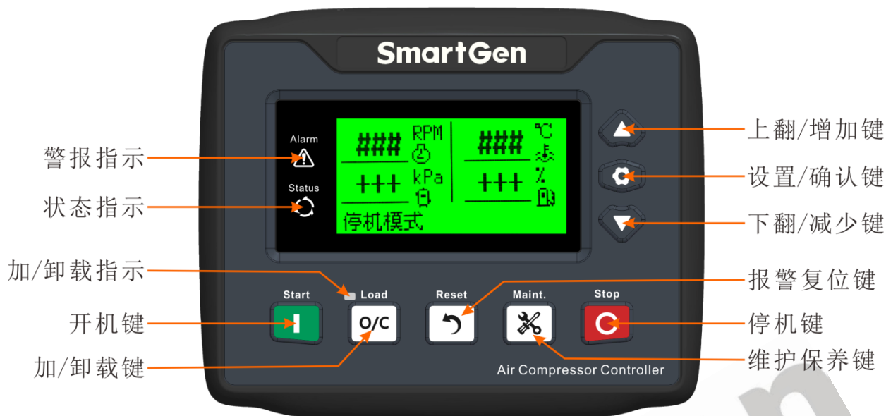
图1 前面板图
