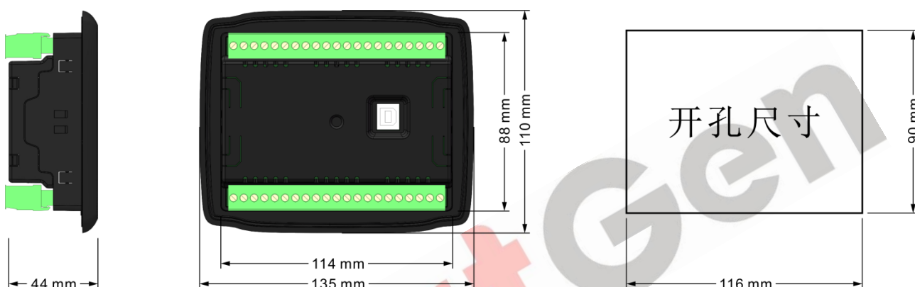
图9 外形及开孔尺寸
